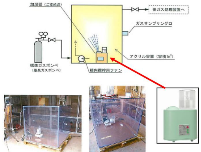
試験装置概略図
